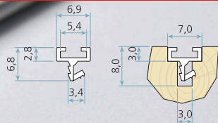
Šířka drážky: 3 mm min. hloubka drážky: 8 mm
