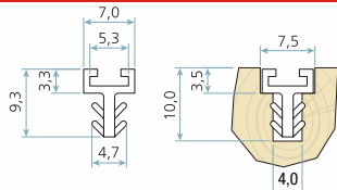
Šířka drážky: 4 mm min. hloubka drážky: 10 mm
