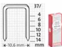
Spony NOVUS typ H 37 - spony z jemného drátu 10,6 x 0,75 mm
