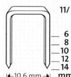
Spony NOVUS typ G 11 - spony z plochého drátu 10,6 x 1,25 mm
