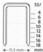
Spony NOVUS typ A 53 - spony z jemného drátu 11,3 x 0,75 mm
