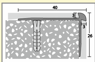
schodová hrana na vruty
