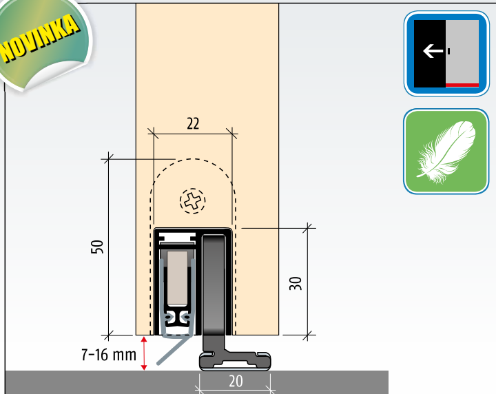
Planet sada vedení - krátká (součást balení) pro spáru 7 - 16 mm - 3 plastová vedení + 1 montážní plech + 2 šrouby
