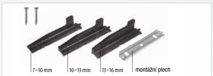
Planet sada vedení - krátká (součást balení) pro spáru 7 - 16 mm - 3 plastová vedení + 1 montážní plech + 2 šrouby
