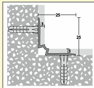
ukončovací profil soklová hrana schodová hrana
