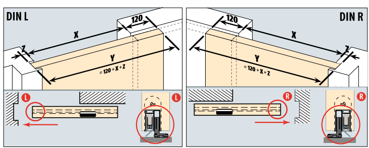
Planet sada vedení - douhá (na objednávku) pro spáru 7 - 16 mm - 3 plastová vedení + 1 montážní plech + 2 šrouby
